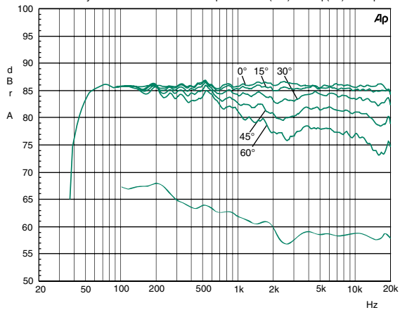
図 5:8320A および 8330A 水平軸の周波数特性。下のカーブはモニターの音響パワーレベルの特性を示している
