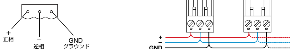
図7. バランス・アナログ入力ユーロブロック入力端子のピン配列 (左) およびユーロブロック入力端子の並列接続 (右)
